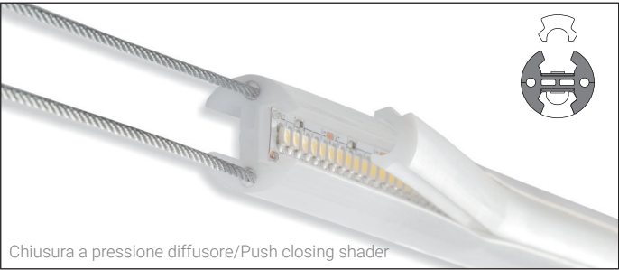
Chiusura a pressione diffusore/ Push closing shaver
